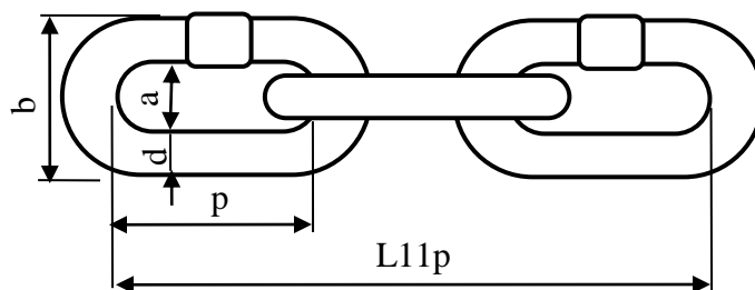
Řetěz dlouhočlánkový
