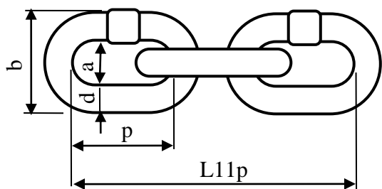
Řetěz krátkočlánkový
